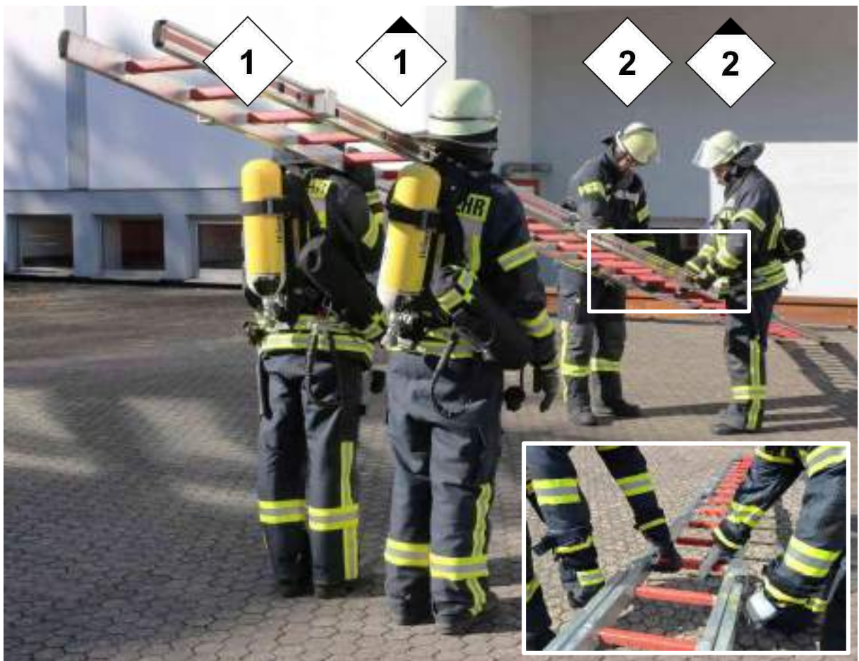
Abbildung 11: Zusammenstecken der Steckleiterteile
