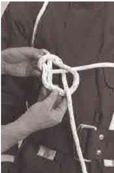
3. Phase – Pfahlstich
