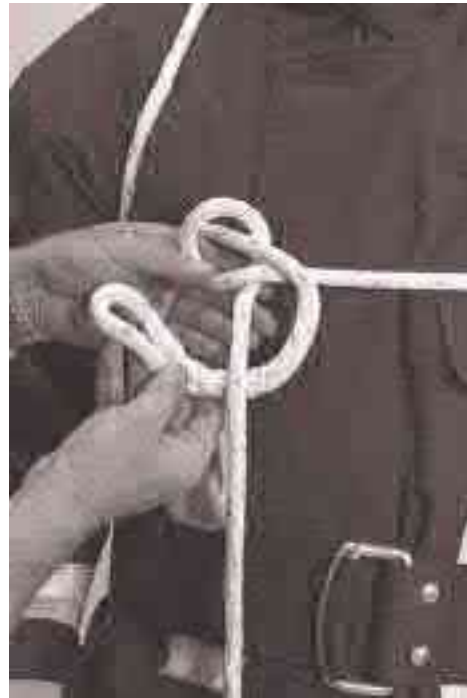
2. Phase – Pfahlstich
